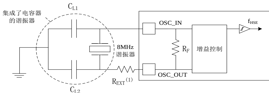
图 15 使用 8MHz 晶体的典型应用
