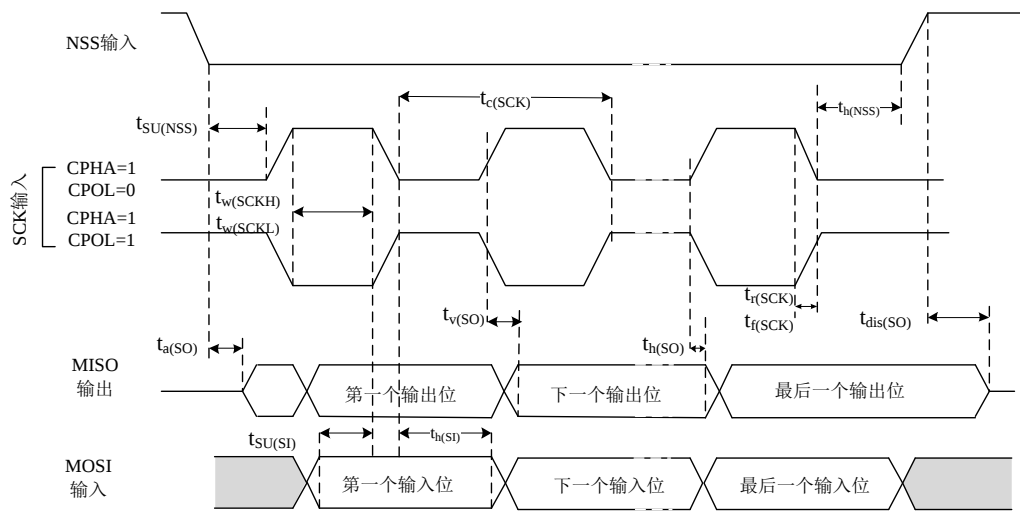
图 27 SPI 时序图- 从模式和 CPHA=1 (1)
