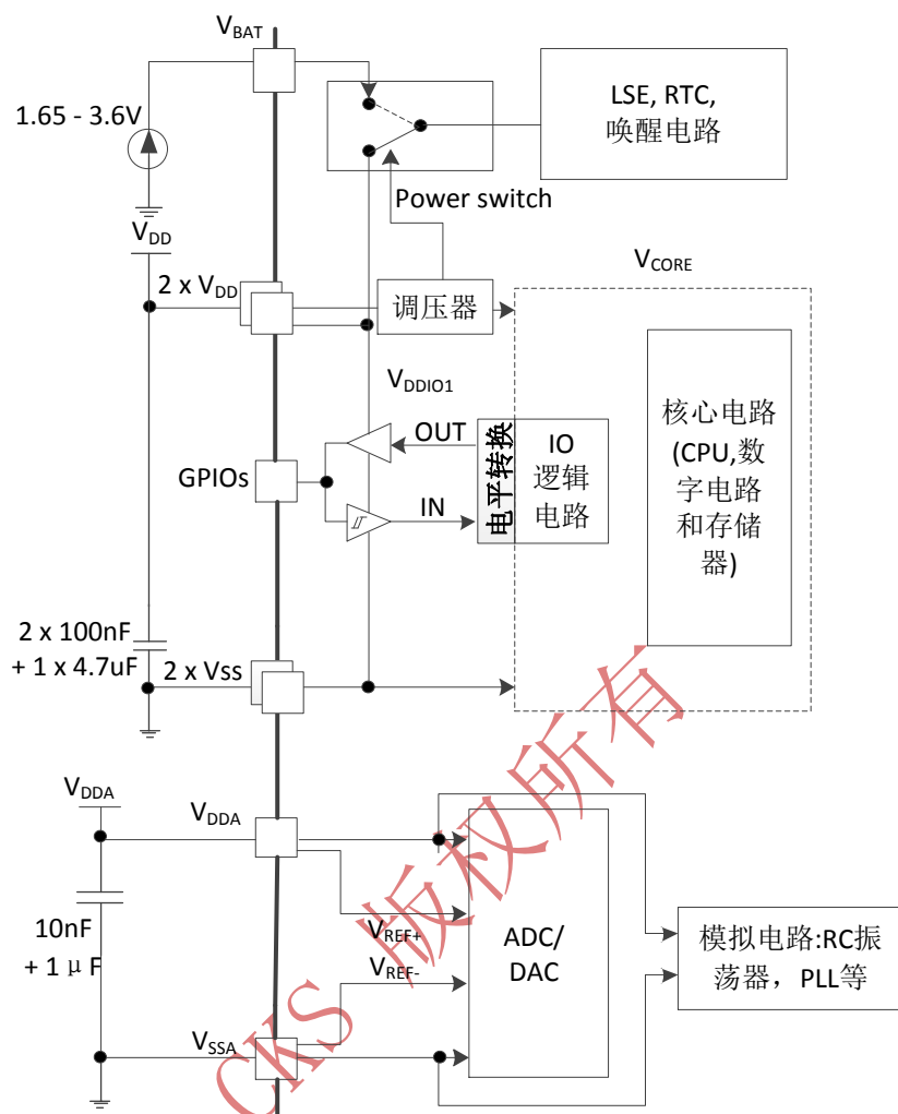
图 11 供电方案
