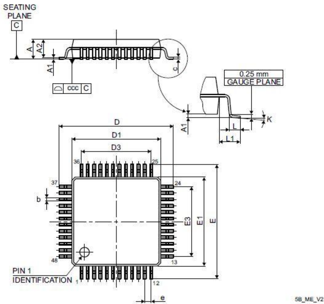
图 33 LQFP48 - 7x7mm 的 48 引脚薄型四方扁平封装外形 (1)
