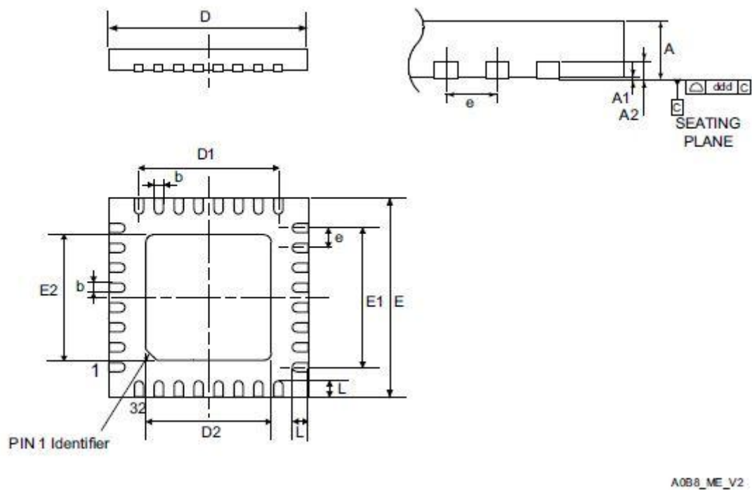
图 39 UFQFPN32 封装外形 (1)
