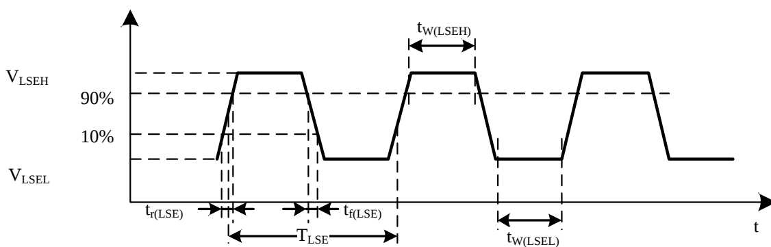
图 14 低速外部时钟源交流时序图
