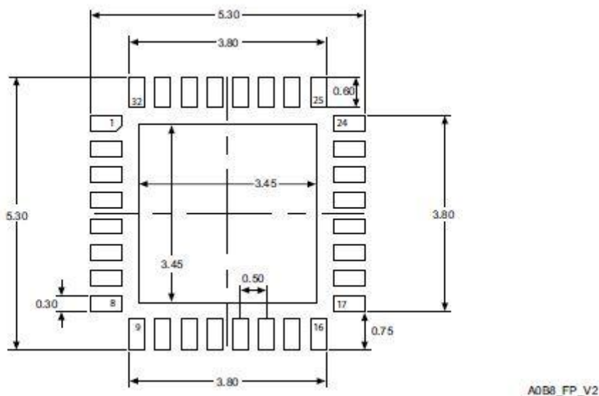
图 40 推荐的 UFQFPN32 封装图
